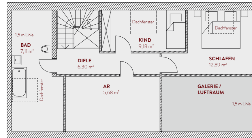
Dachgeschoss (obere Ebene)
